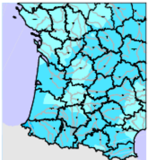
B1 - 2050
