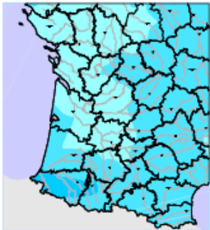
B1 - 2050
