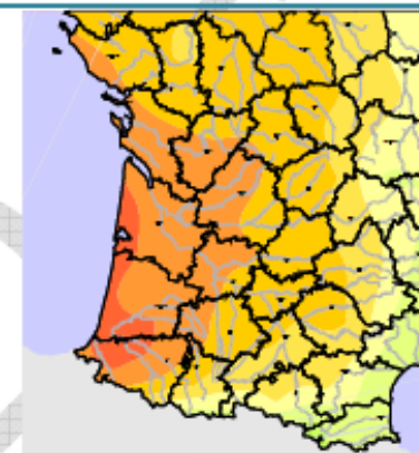
A1B – 2080
