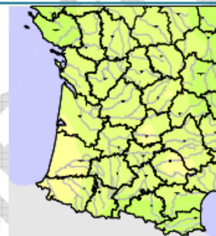
A2 - 2050
