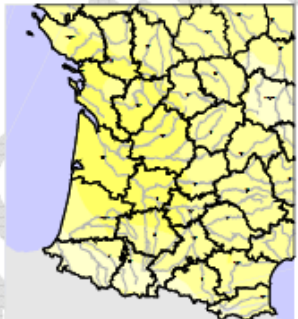
A2 - 2050
