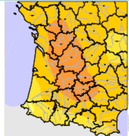
A1B - 2050
